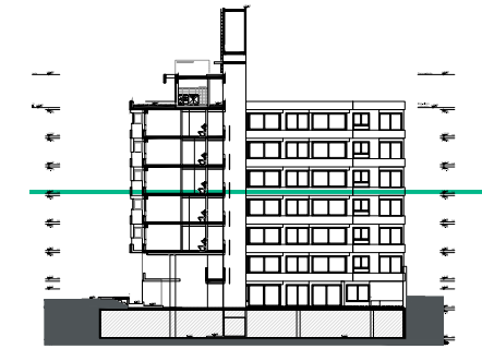
Corte A-A
