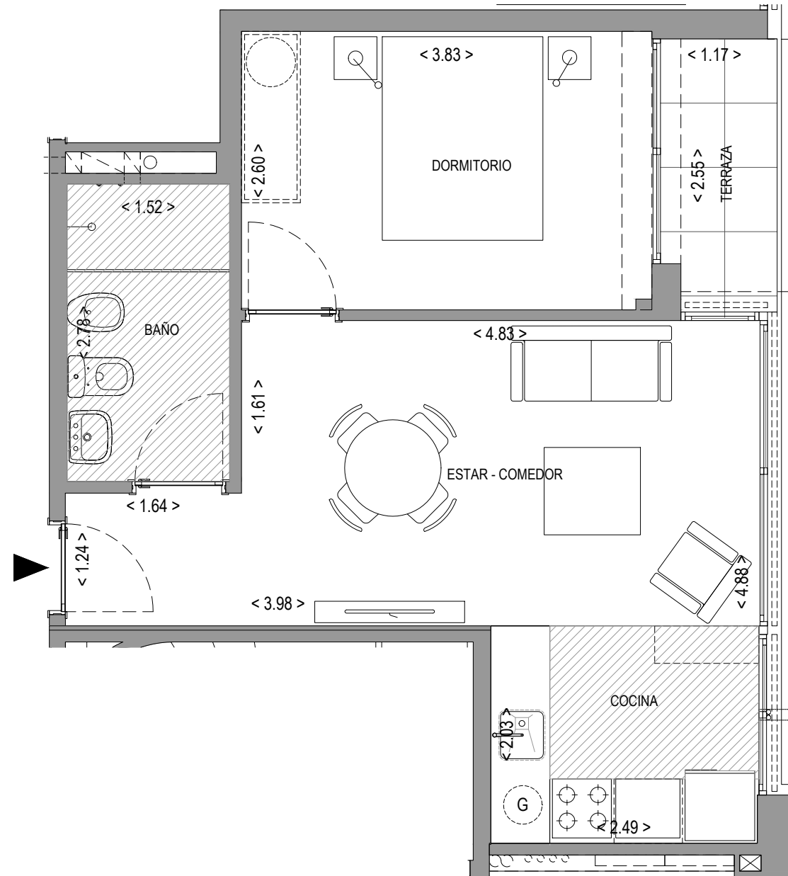
Planta Esc: 1/50
