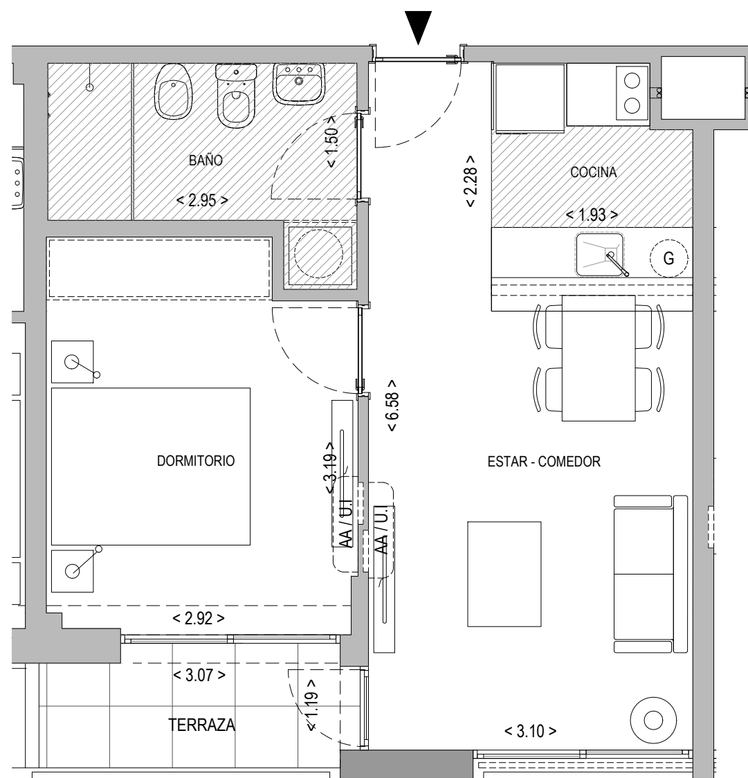
Planta Esc: 1/50
