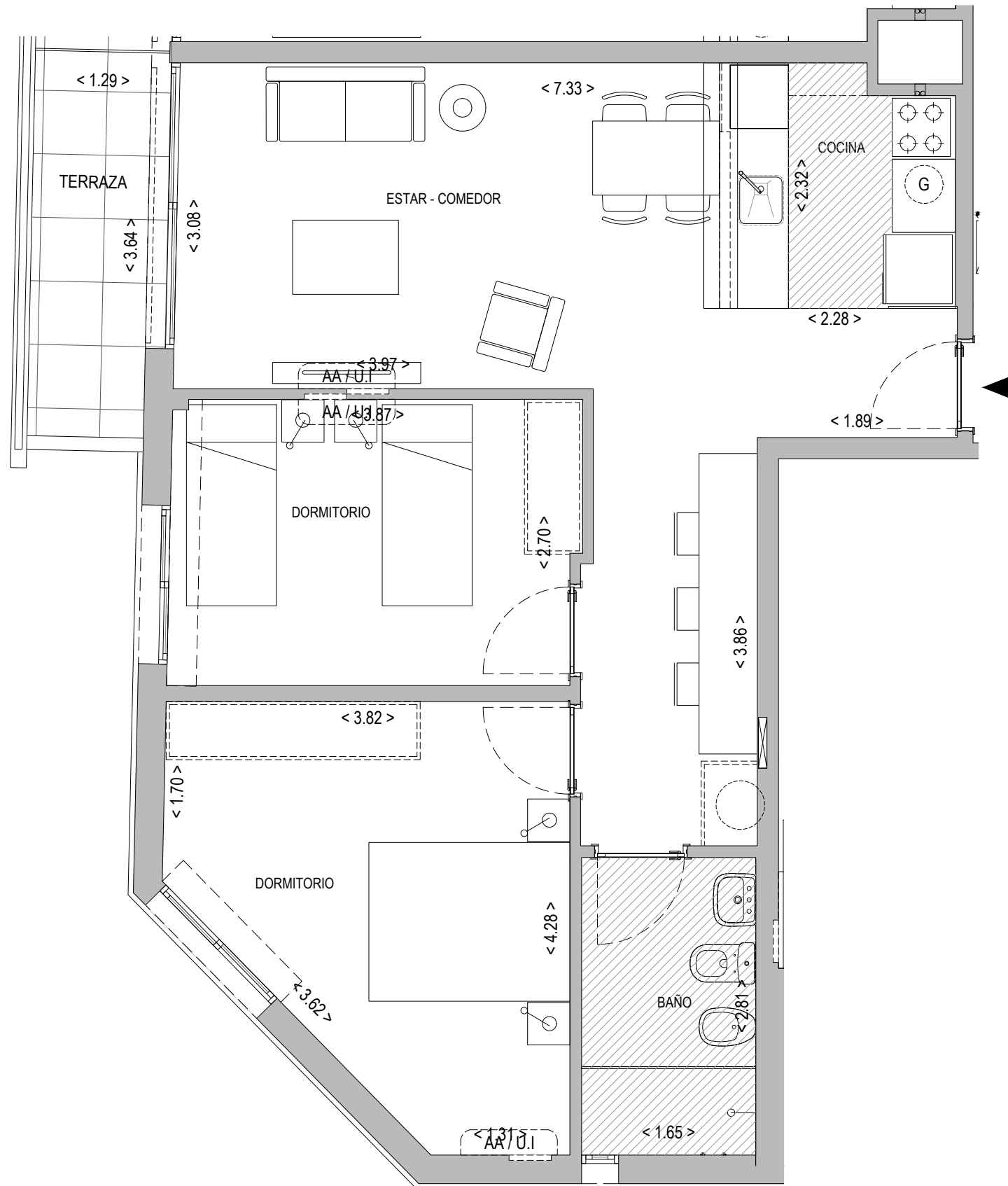
Planta Esc: 1/50
