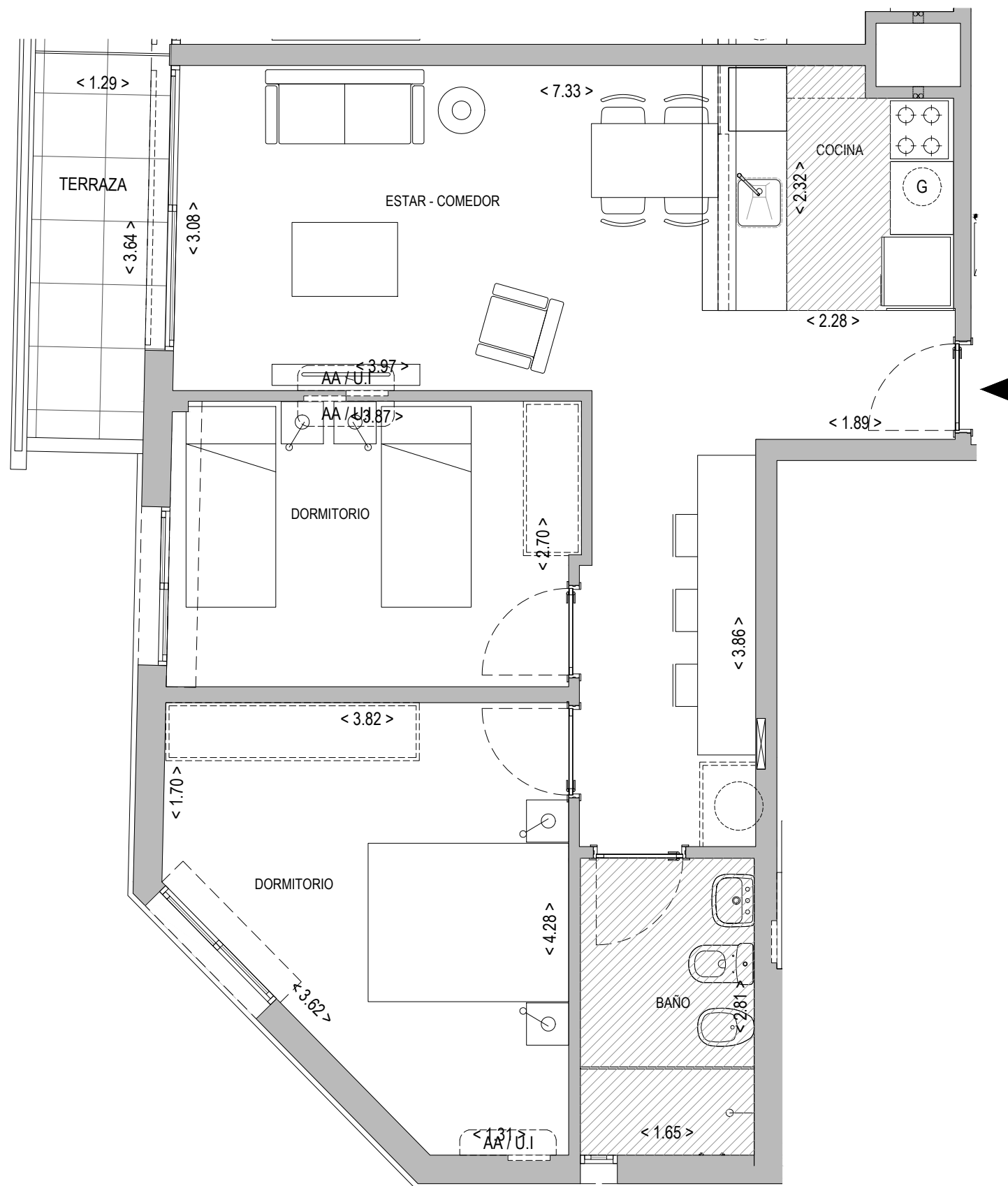
Planta Esc: 1/50
