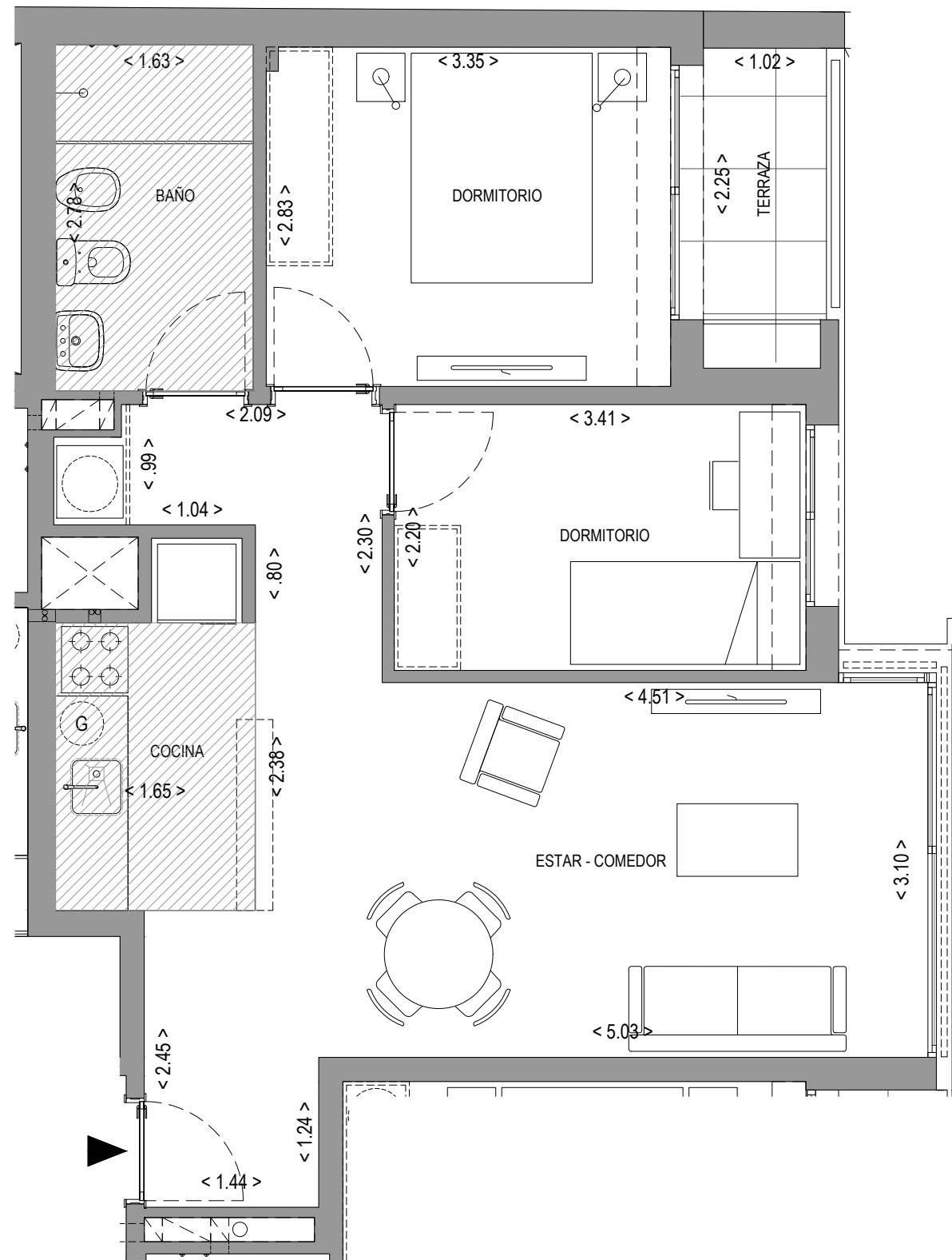
Planta Esc: 1/50
