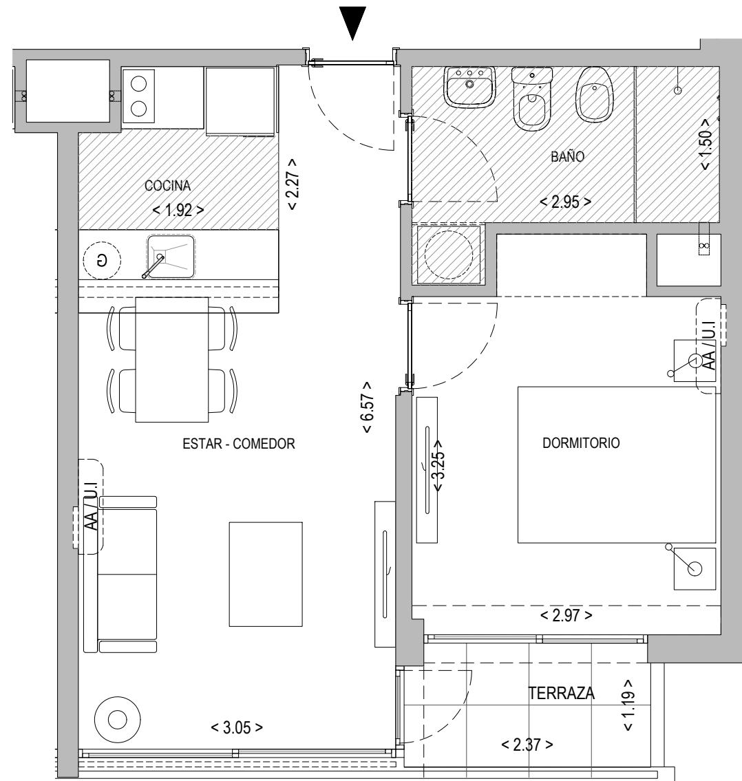
Planta Esc: 1/50
