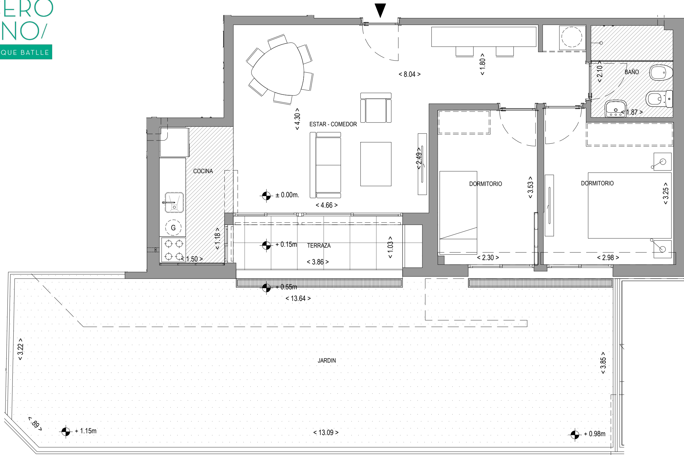
Planta Esc: 1/50
